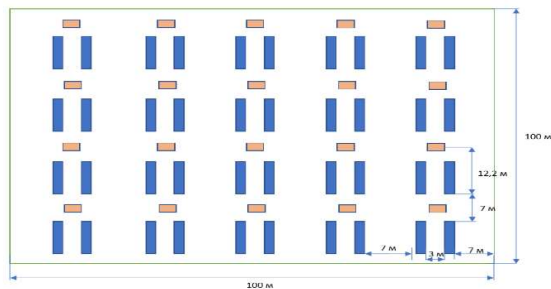
Схема расстановки контейнеров на площадке.
